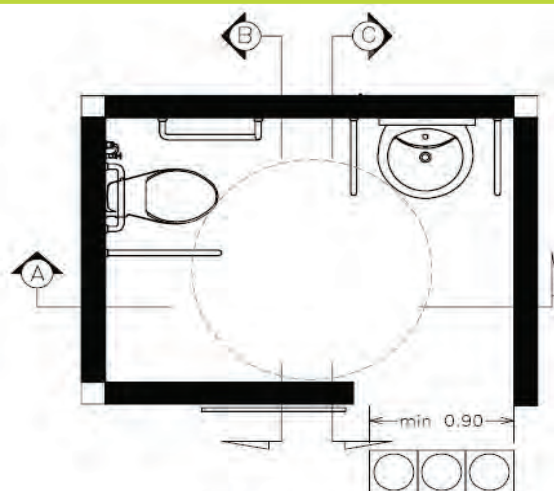
ผังพื้นห้องน้ำคนพิการ ประเภท B มาตราส่วน 1 : 50
