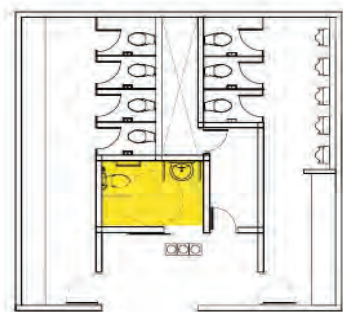
ผังพื้นห้องน้ำ ประเภท B มาตราส่วน 1 : 50
